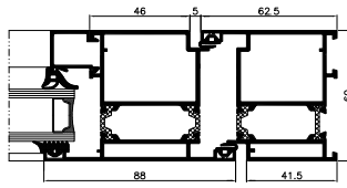
przekrój drzwi
